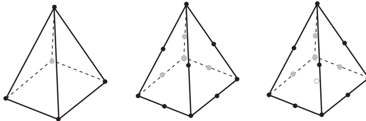
(d) 5-, 13-, and 14-pyramid elements (CPYRAM)
