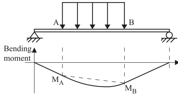
a) Actual beam structure bending moment diagram
